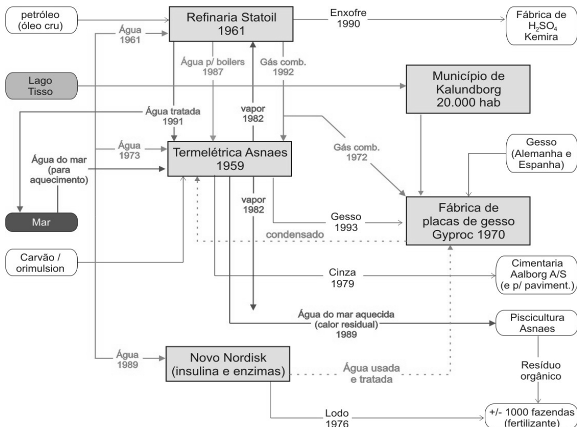
Figura 3 - Fluxograma da simbiose industrial em Kalundborg
